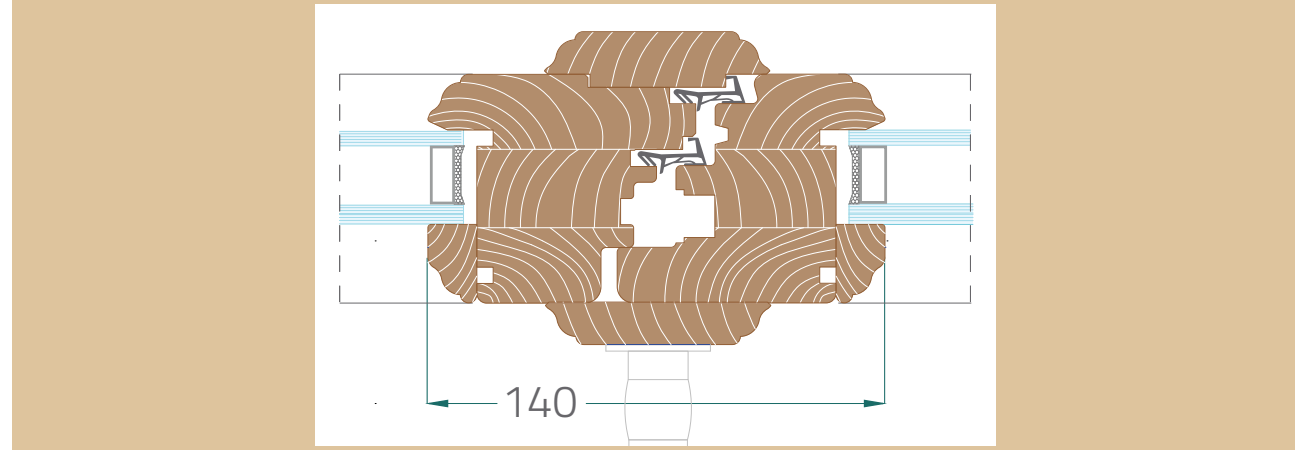
NODO RIDOTTO CON ENTRATA "ZERO" E PROFILO BAROCCO I/E
