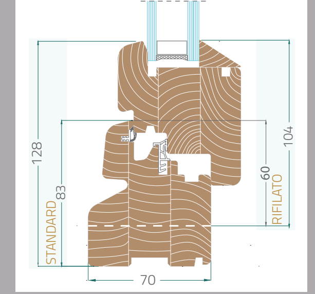
SEZIONE NODO INFERIORE IN LEGNO
