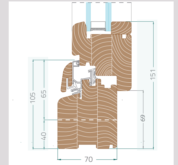
SEZIONE NODO INFERIORE IN ALLUMINIO
