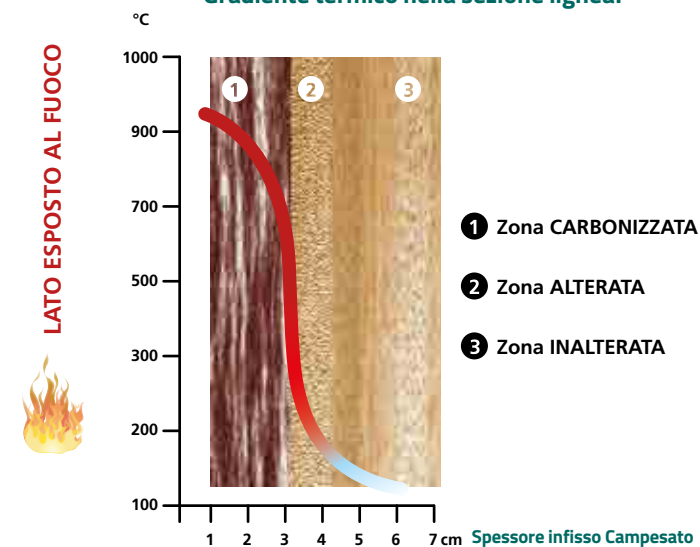
Gradiente termico nella sezione lignea.
