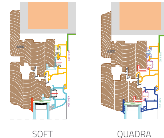
Soluzioni con coprifilo complanare per il serramento legno/alluminio
