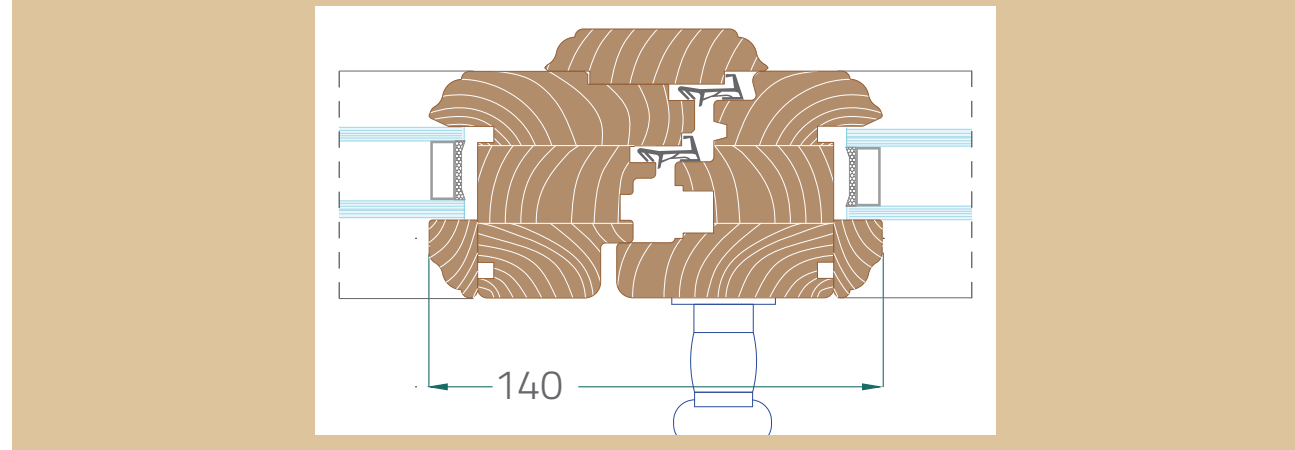
NODO RIDOTTO CON PROFILO BAROCCO I/E
